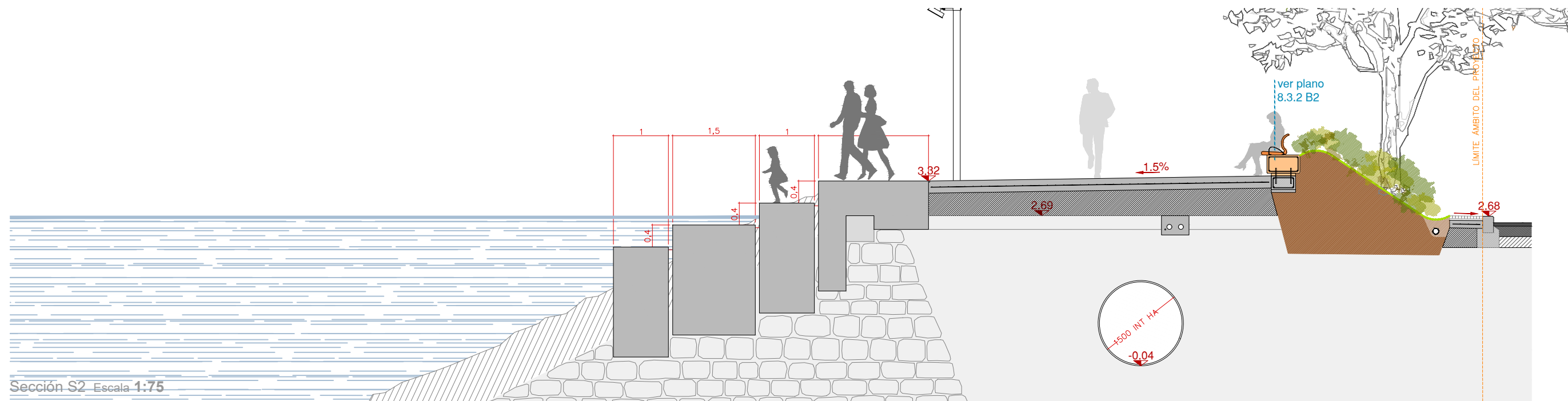
Sección S1 Escala 1:75
