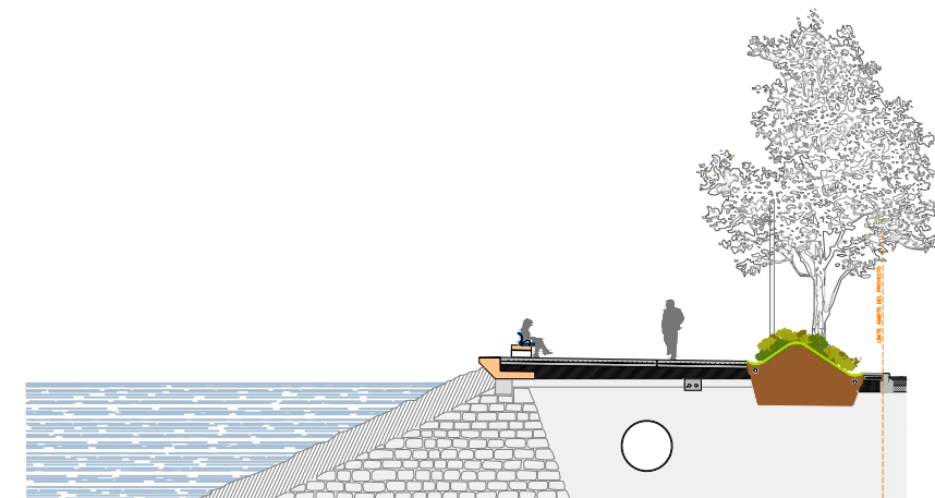
Sección S3 Escala 1:250
