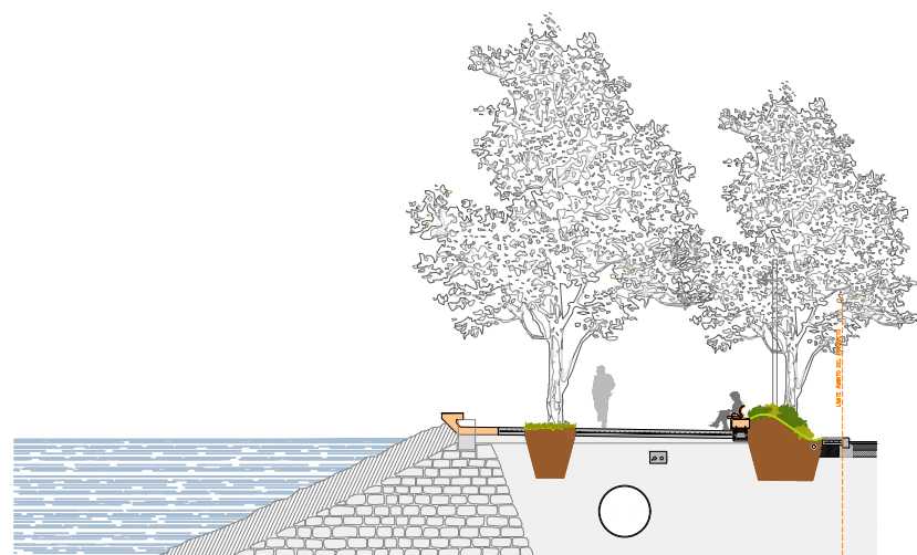
Sección S1 Escala 1:250
