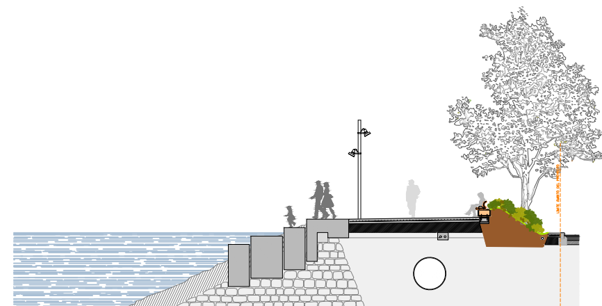
Sección S2 Escala 1:250
