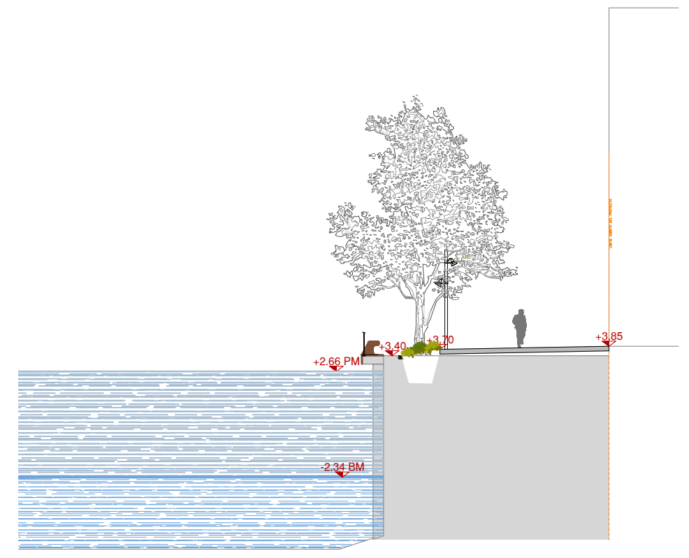
Sección 1 Escala 1:250
