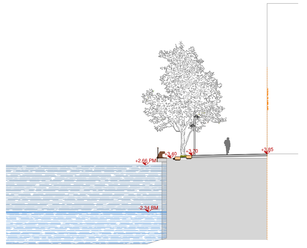
Sección 2 Escala 1:250
