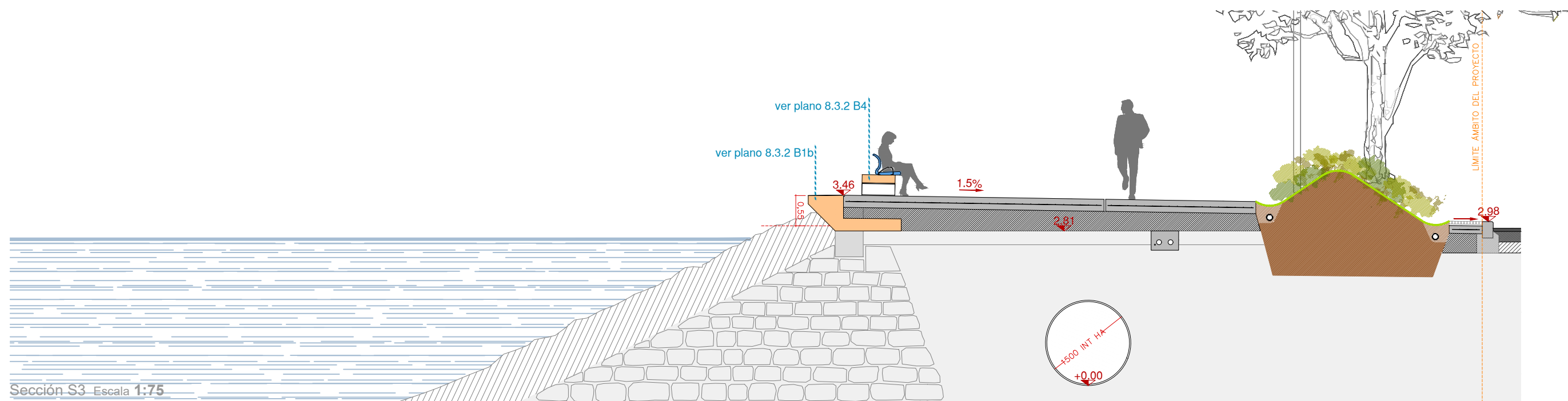
Sección S2 Escala 1:75
